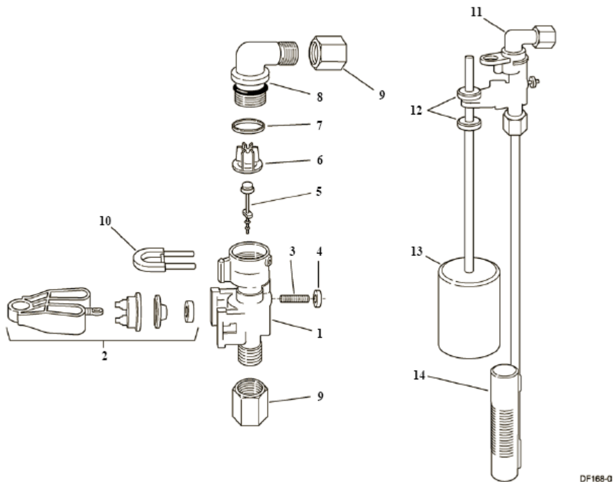
Рис. 21: Предохранительный рассольный клапан 2310
