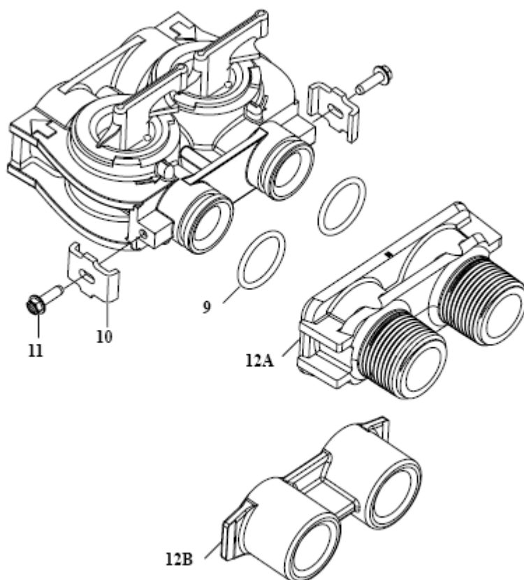
Рис. 18: Узел переливного клапана, пластмасса
